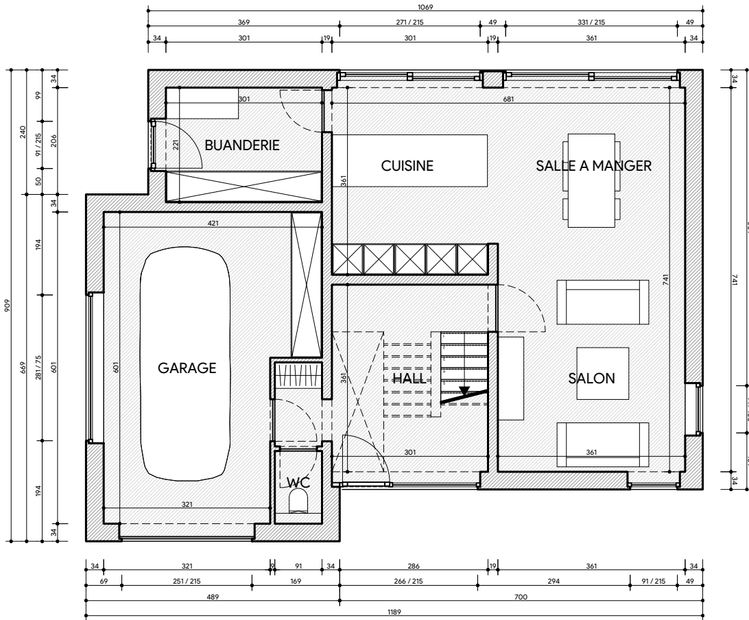
REZ-DE-CHAUSSEE ECH. 1/100
