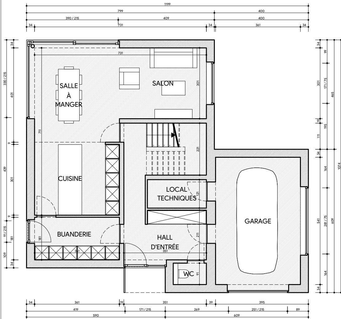
REZ-DE-CHAUSSEE ECH. 1/100
