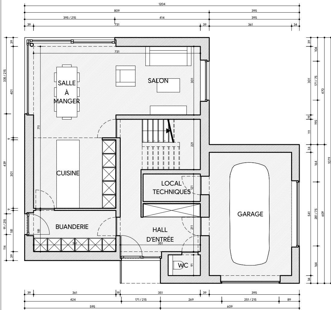
REZ-DE-CHAUSSEE ECH. 1/100
