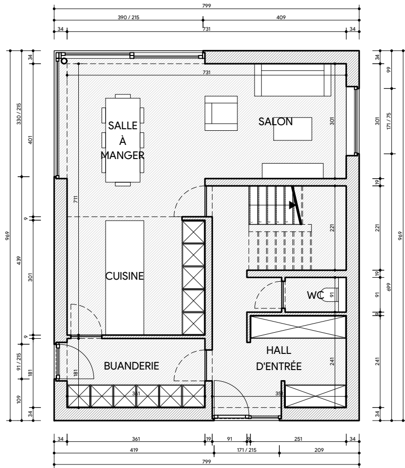
REZ-DE-CHAUSSEE ECH. 1/100
