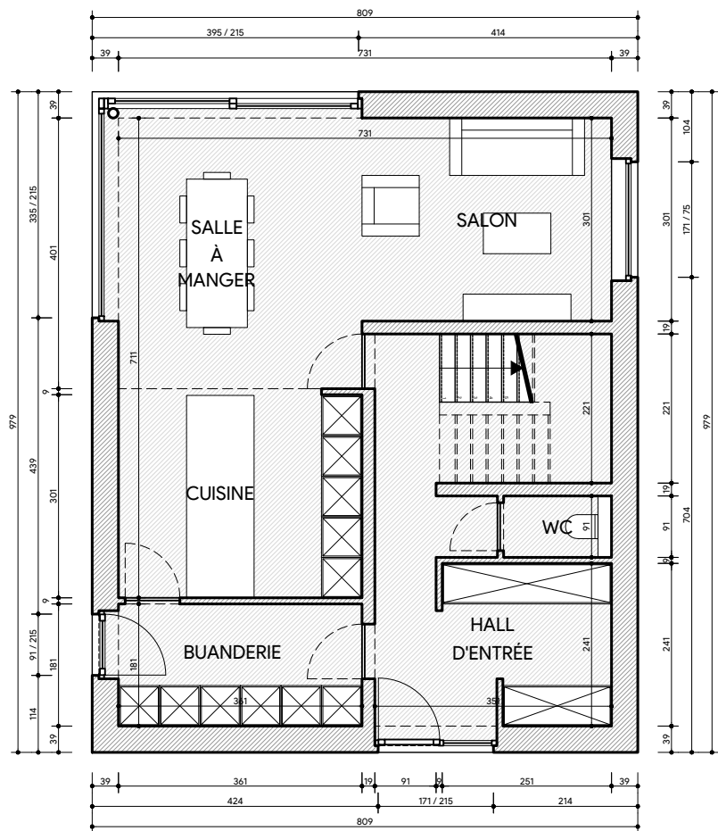
REZ-DE-CHAUSSEE ECH. 1/100
