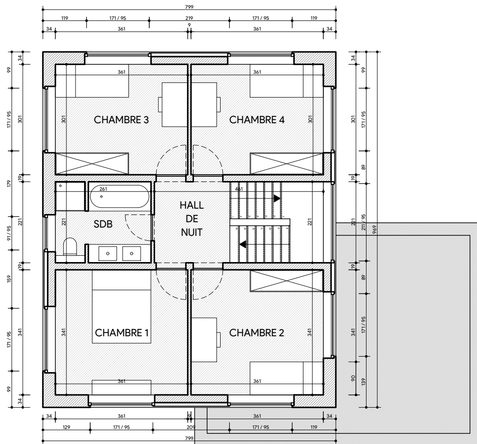
PREMIER ETAGE ECH. 1/100
